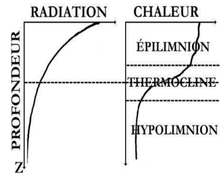
Distribution verticale du rayonnement lumineux et de la chaleur dans un lac stratifié (d'après U. Lemmin, 1995)
