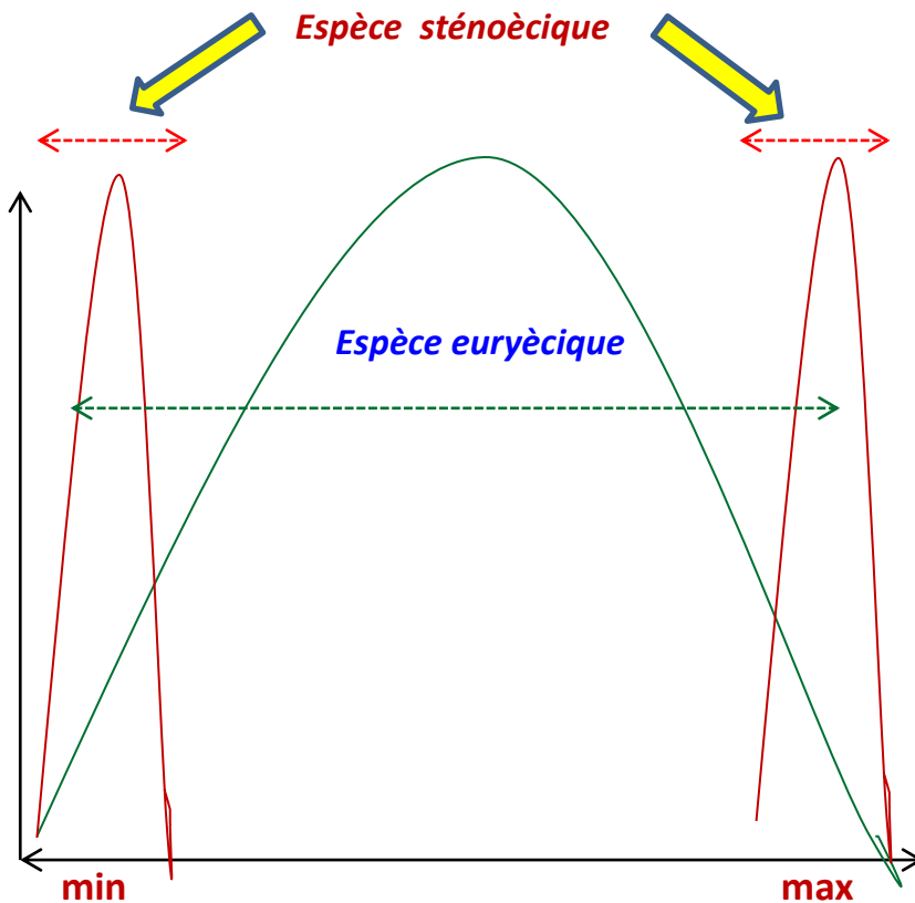
Courbe C1 de Shelford
